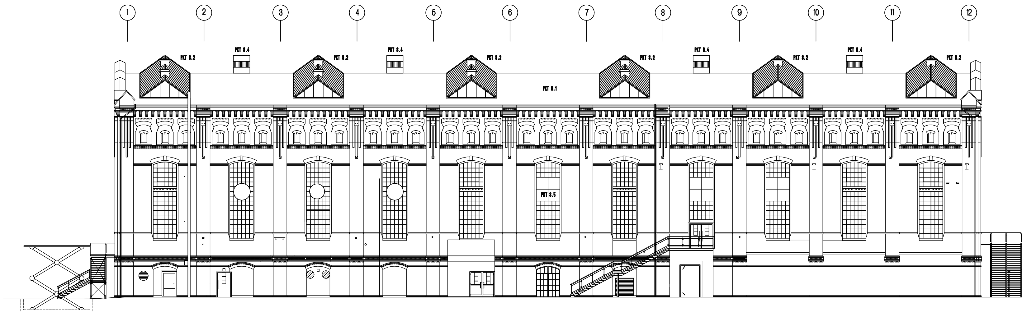
Ansicht Nordost
