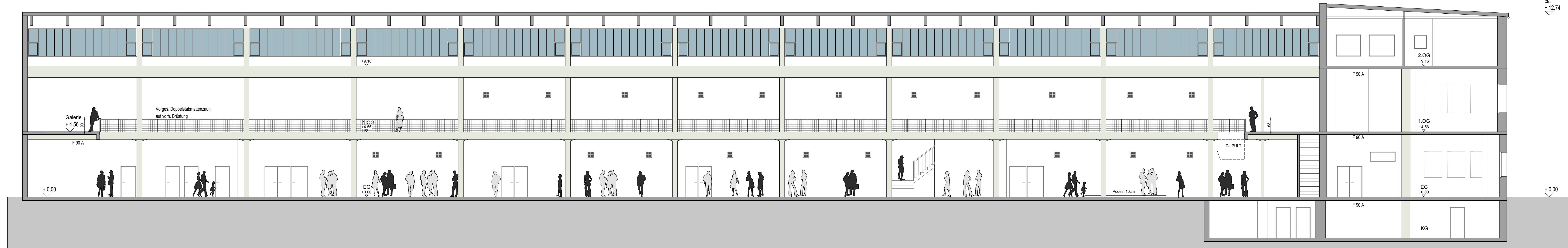
SYSTEMSCHNITT B-B
