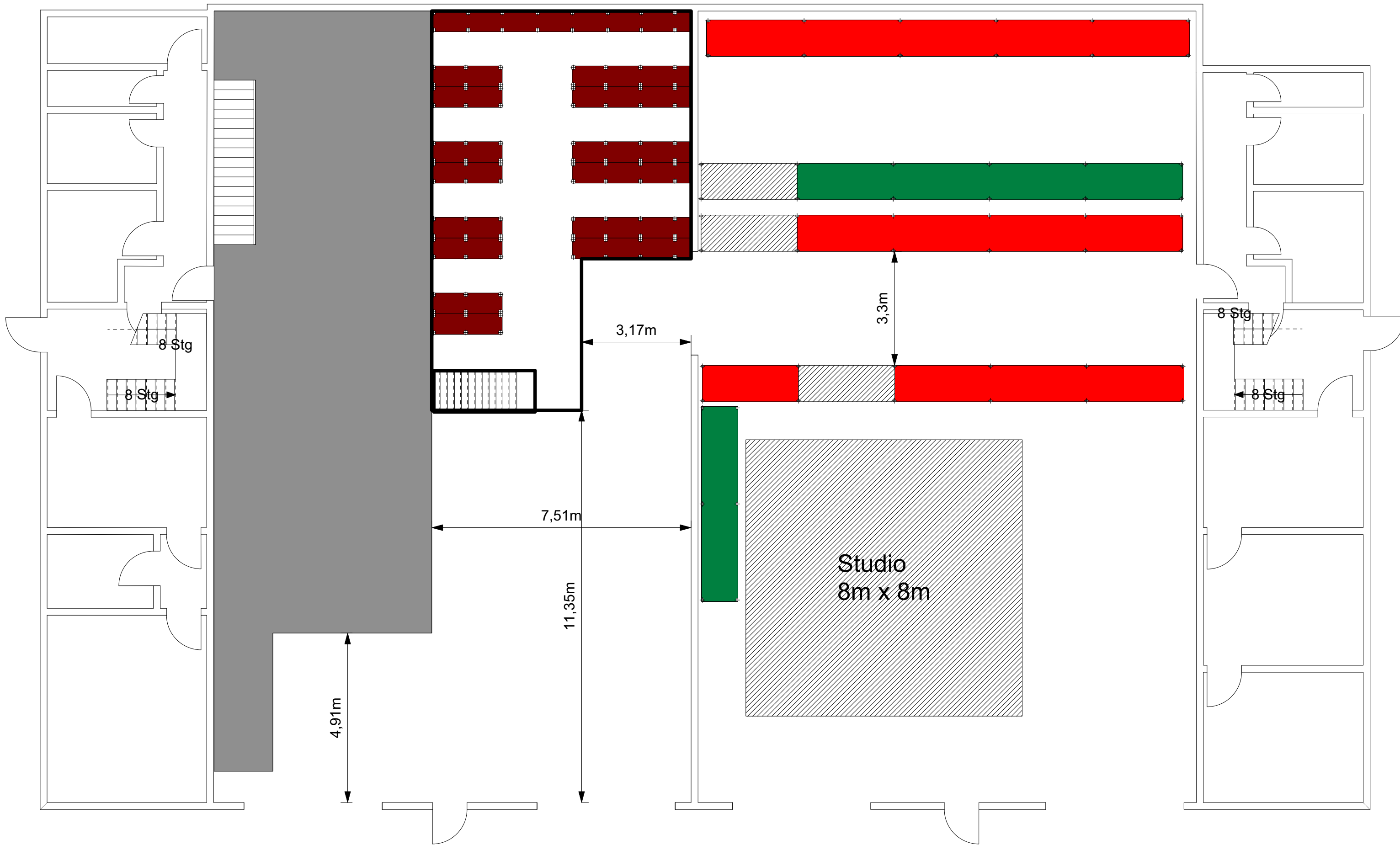
Erdgeschoss 1:100
