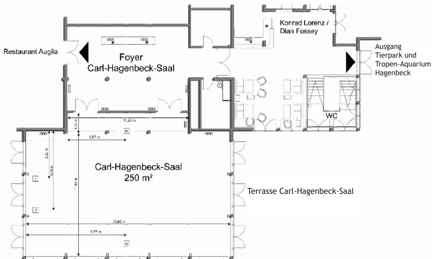
Carl-Hagenbeck-Saal Grundriss; das Bild zeigt die Eingänge des Saals.
