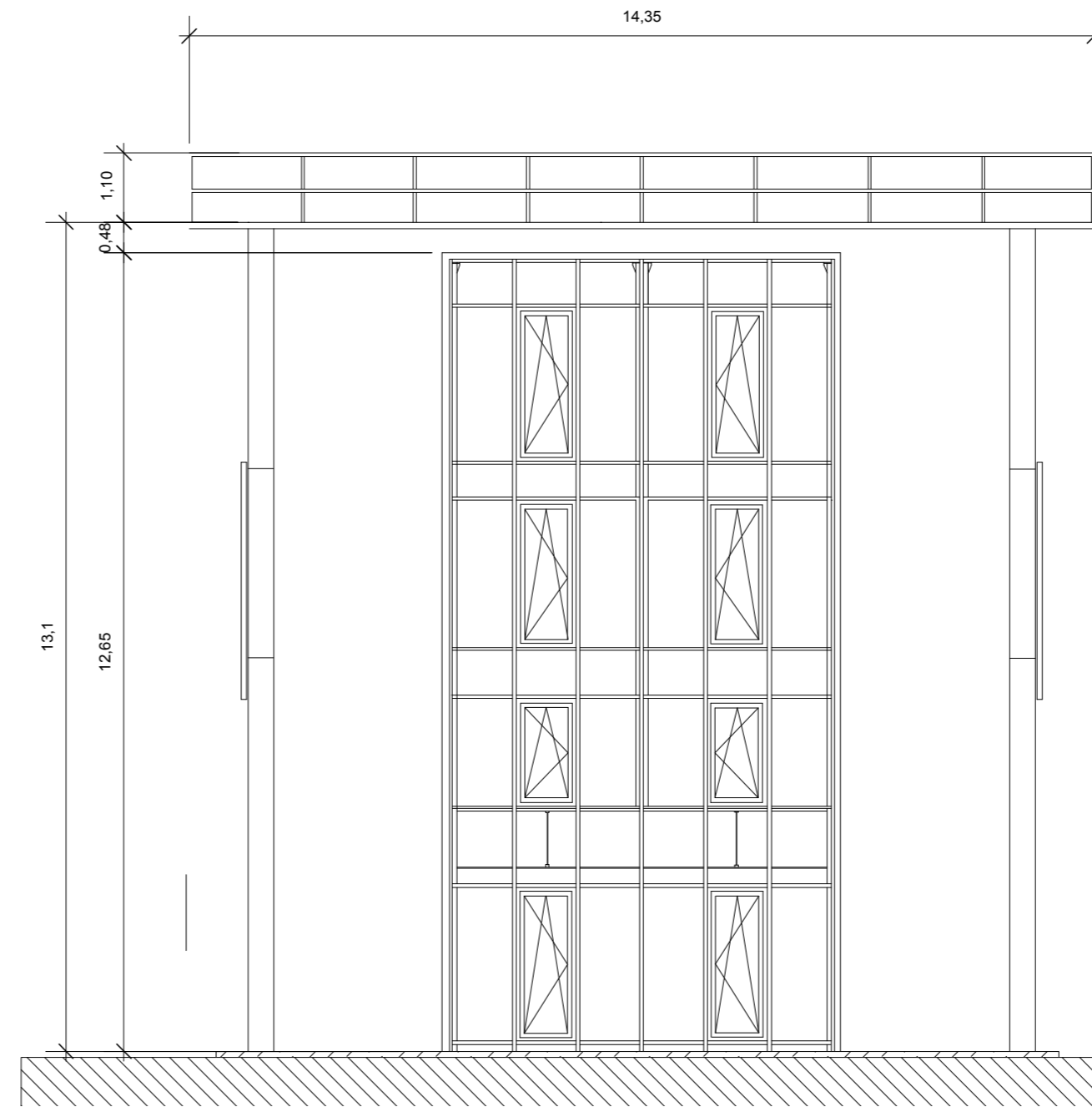
Südansicht (Spreeseite)
