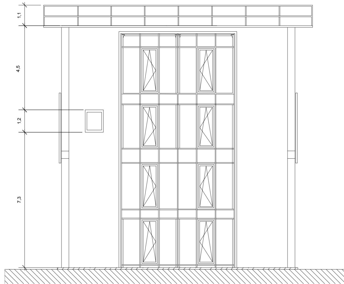
Nordansicht (Straßenansicht)
