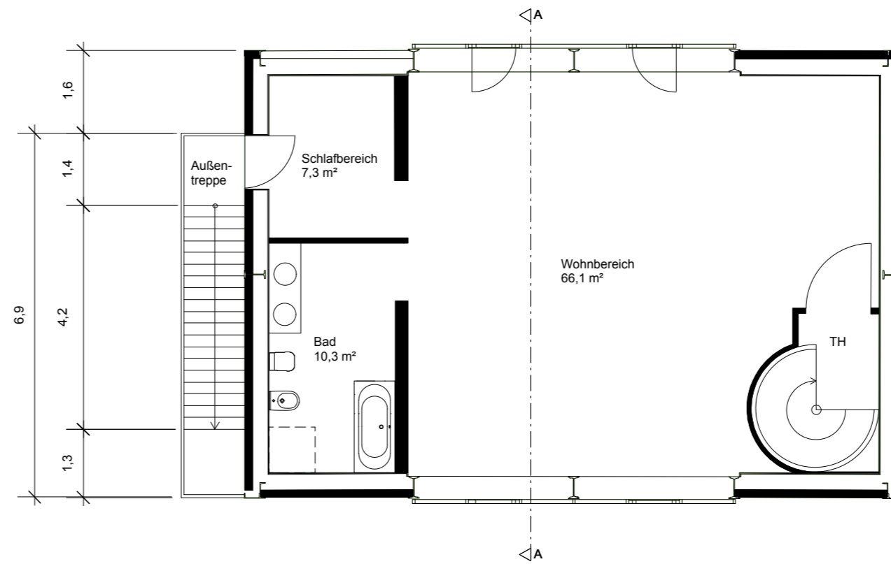
Betriebsinhaberwohnung 3.OG
