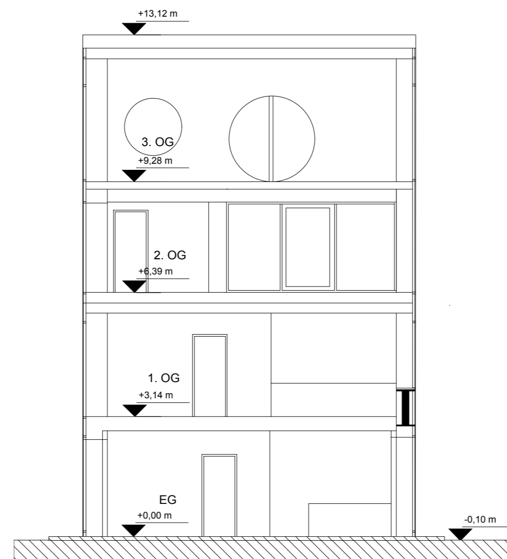
Schnitt AA
