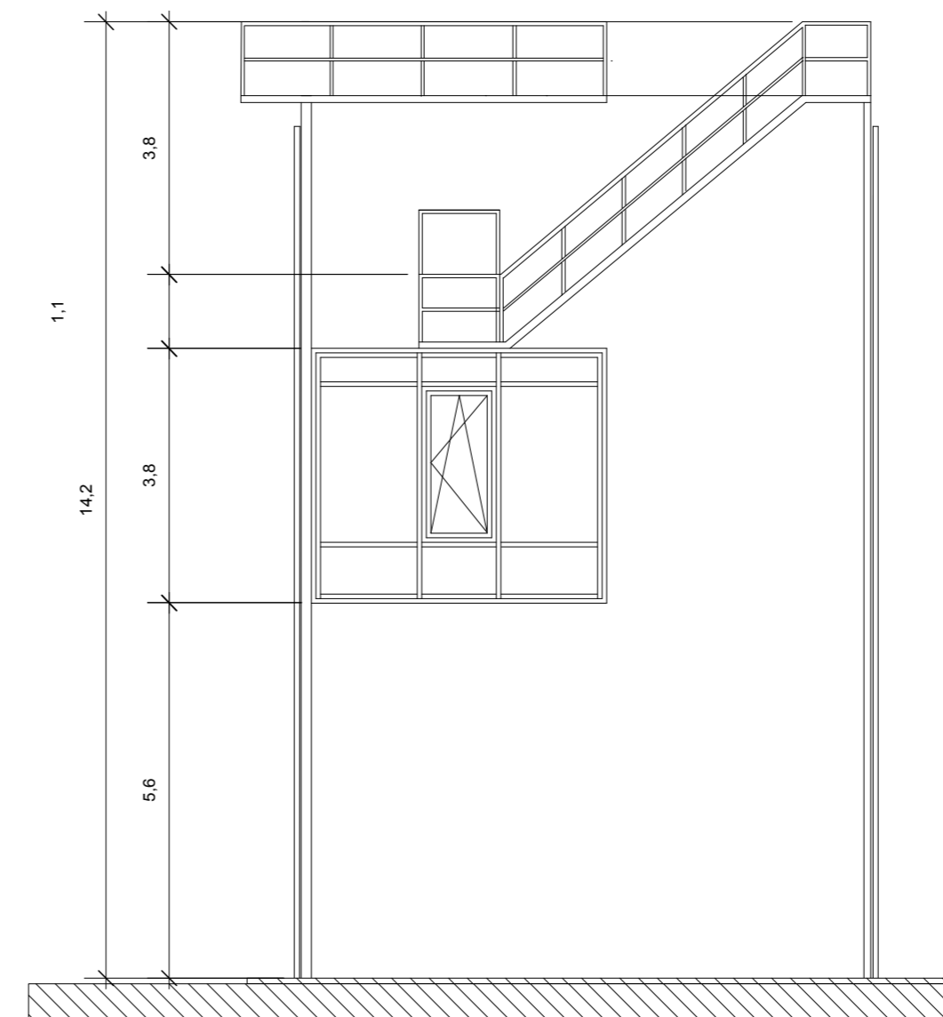
Ostansicht
