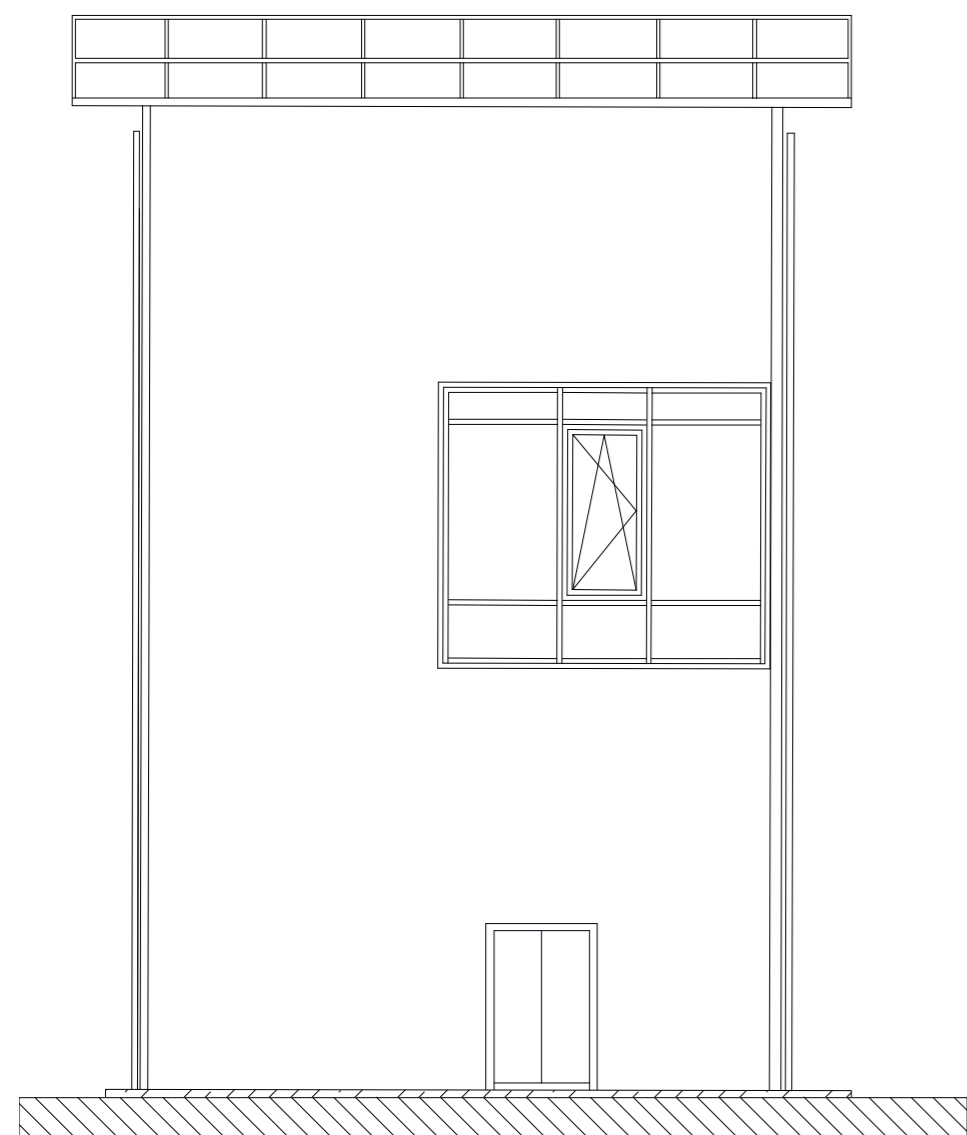
Westansicht
